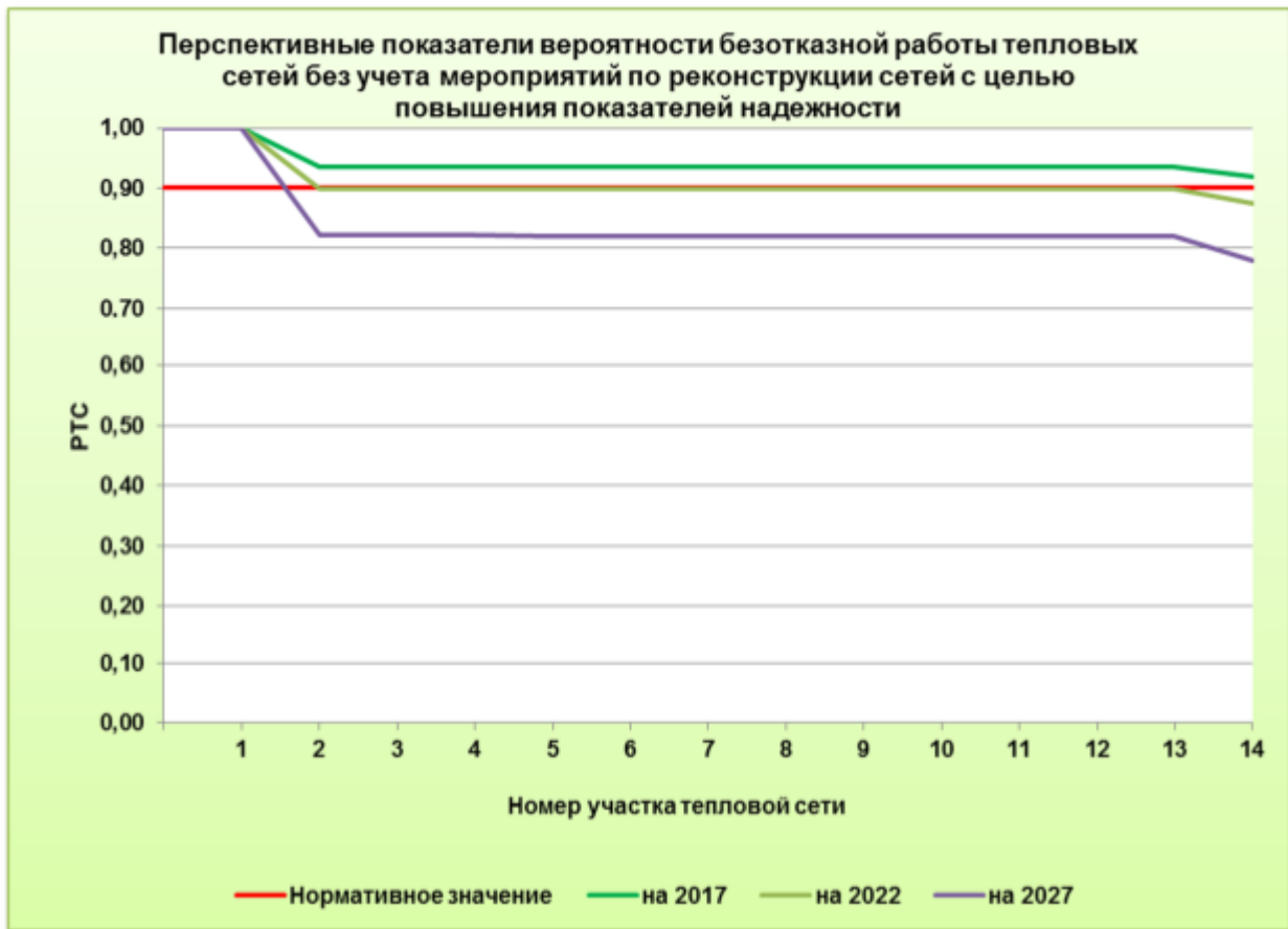
Рисунок 3.9 Вероятность безотказной работы тепловых сетей от Архангельской ТЭЦ до ТК-18т-4
