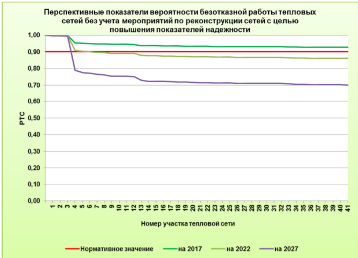
Рисунок 3.4 Вероятность безотказной работы тепловых сетей от 55-7а до 55-19-16-2
