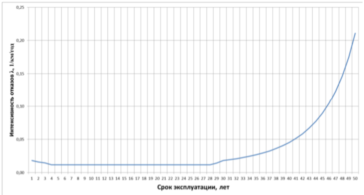
Рисунок 2.1 – Зависимость интенсивности отказов от срока эксплуатации участка тепловой сети для систем теплоснабжения города Архангельска.
